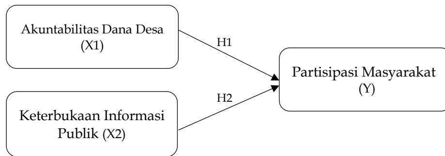
Gambar 1. Kerangka Penelitian
